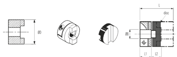
Tabulka 10.9 Rozměry hřídelových spojek pro lineární osy KK
